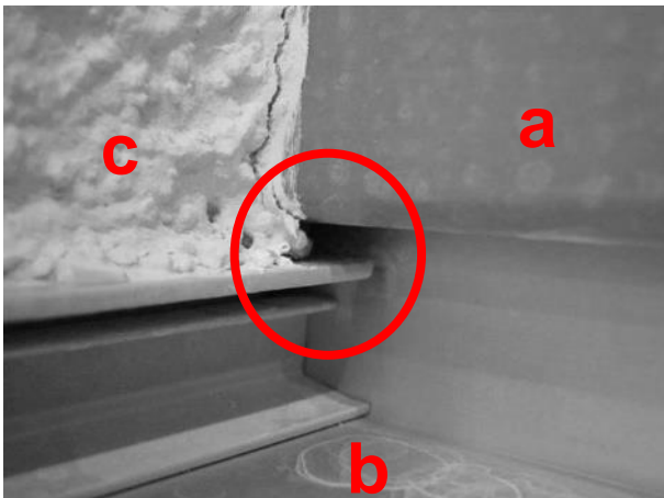
Abbildung 2: Beispiel für ein Gewerke Loch im Eckbereich zwischen Fensterrahmen (a), Fensterbank (b) und Fassade / Laibung (c)
