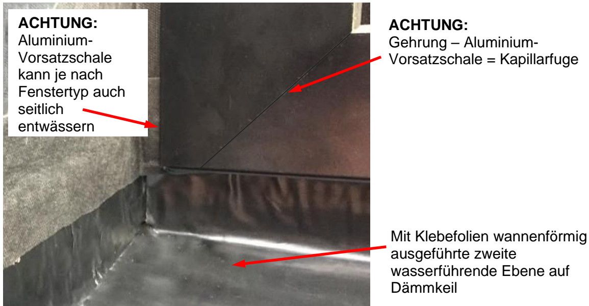
Abbildung 15: Die zweite wasserführende Ebene hintergreift die Aluminium-Vorsatzschale des Fensters und gewährleistet somit, dass etwaig anfallendes Wasser (Entwässerung, Kapillarfuge Gehrung, Gewerke Loch) auf dieser nach vorne abgeleitet werden kann (Abbildung noch ohne Fensterbank und noch ohne Laibung).
