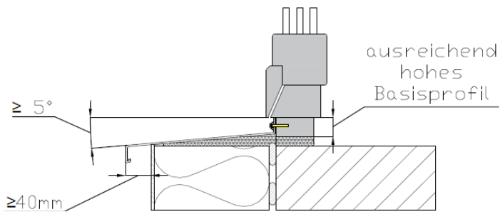
Abbildung 12: Fensterbankanschluss mit ausreichend hohem Fensterbankanschlussprofil mit mind. 5° Fensterbankneigung und einem Fensterbankvorsprung von mind. 40 mm
