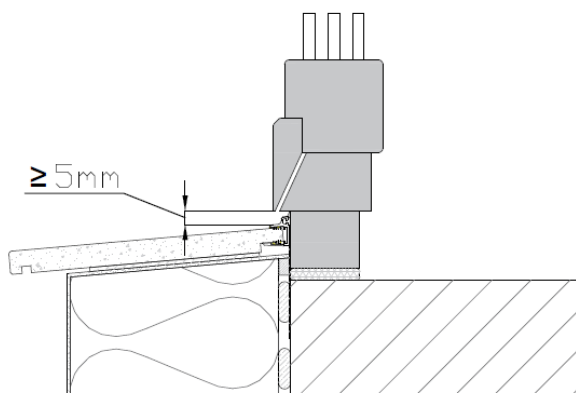
Abbildung 14: Darstellung eines ausreichend hohen Abstands zur gesicherten Wasserabführung
