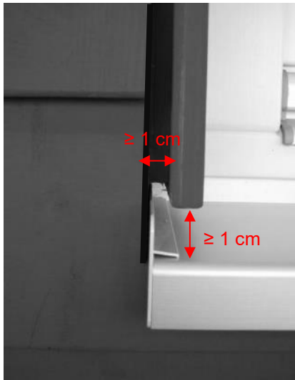
Abbildung 29: Laibungsbrett mit ausreichendem Abstand ( \geq 1 cm) zur Fassadenschalung und zur Fensterbankfläche (Quelle: Holzforschung Austria)
