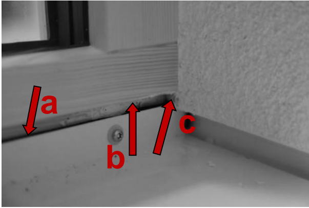
Abbildung 19: ordnungsgemäßer Einbau einer Fensterbank (a) eingebautes Fugendichtband (b) verschlossene Fensterrahmennut mittels Dichtmasse (c) geschlossenes Gewerke Loch mittels Dichtmasse
