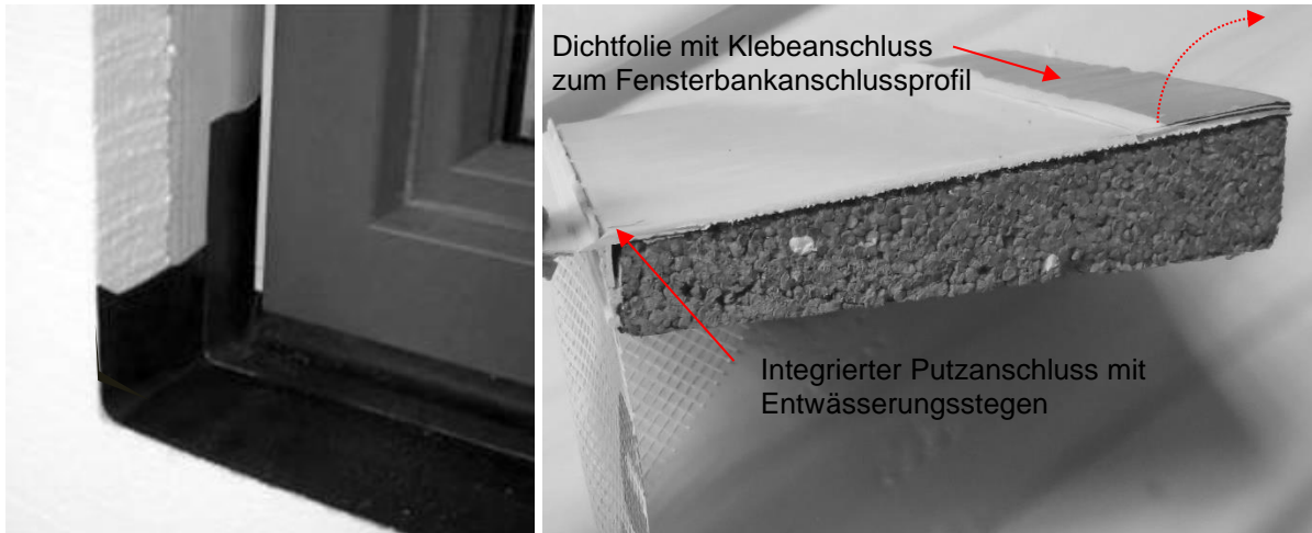
Abbildung 27: Ausführungen mit Klebefolien bei vorgefertigten Holzrahmenelementen im Werk; Folien werden wannenförmig auf Dämmkeil ausgeführt, danach erfolgt die Montage der Fensterbank. Die Laibungsplatten werden im Anschluss mit vorkomprimierten Dichtbändern auf die Endprofile gesetzt; rechtes Bild zeigt einen Dämmkeil mit Dichtfolie und integriertem vorderen Putzanschluss mit definierten Entwässerungsstegen, wie er im vorgefertigten Holzbau Verwendung findet.
