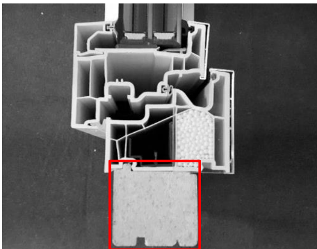
Abbildung 13: Beispiel für ein Fenster mit einem ausreichend hohen, ebenen und dämmenden Fensterbankanschlußprofil (roter Rahmen)
