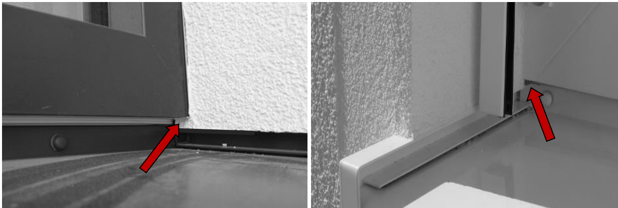
Abbildung 17: Bei nicht eingeputzten Führungsschienen oder bei Einbau ohne Führungsschienen entsteht das Gewerkeloch in der Regel im Zuge der Fassadenarbeiten und ist daher durch den Fassadenhersteller zu schließen.
