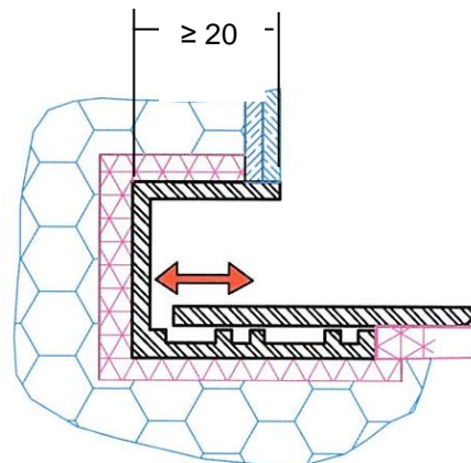
Abbildung 24: eingeputztes Gleitendstück in dem sich die Fensterbank bewegt - Beispiel und Prinzipskizze
