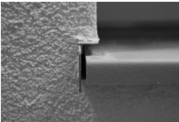
Abbildung 24: eingeputztes Gleitendstück in dem sich die Fensterbank bewegt - Beispiel und Prinzipskizze
