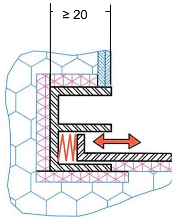
Abbildung 23: eingeputztes Gleitabschlussprofil mit federnder Wirkung - Beispiel und Prinzipskizze
