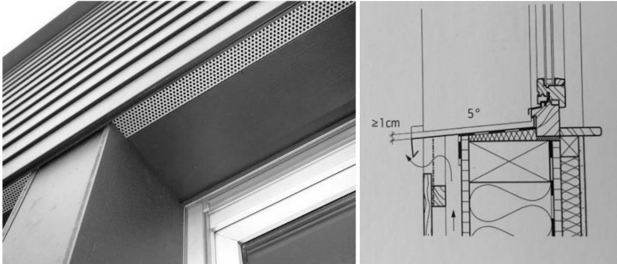
Abbildung 28: Zu- und Abluftöffnungen bei hinterlüfteter Fassade (Quelle: Fassaden aus Holz; proHolz Austria, Holzforschung Austria)
