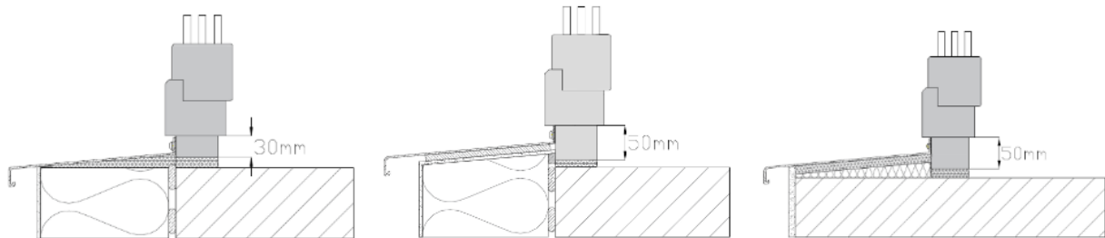
Abbildung 5: schematische Darstellung möglicher Fensteranschlussprofilhöhen (links: Montage während der Fassadenarbeiten – FB eingeputzt; Mitte: nachträgliche Montage Fensterbank – WDVS an Basisprofil angeschlossen; rechts: monolithisches Mauerwerk)
