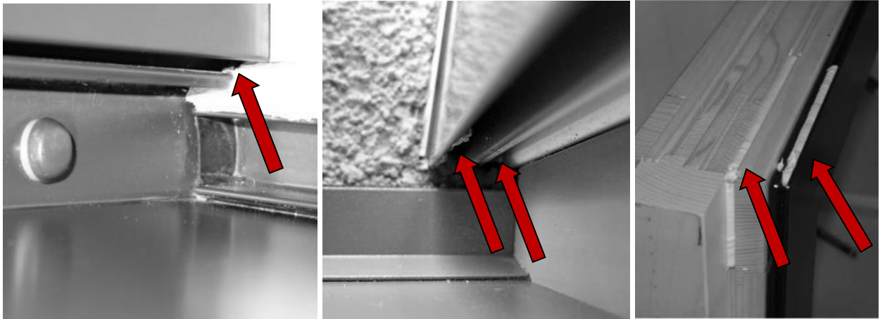
Abbildung 16: Fensterrahmennuten / Vorsatzschalennuten; Verschließen der Nuten mittels z.B. Dichtmasse
