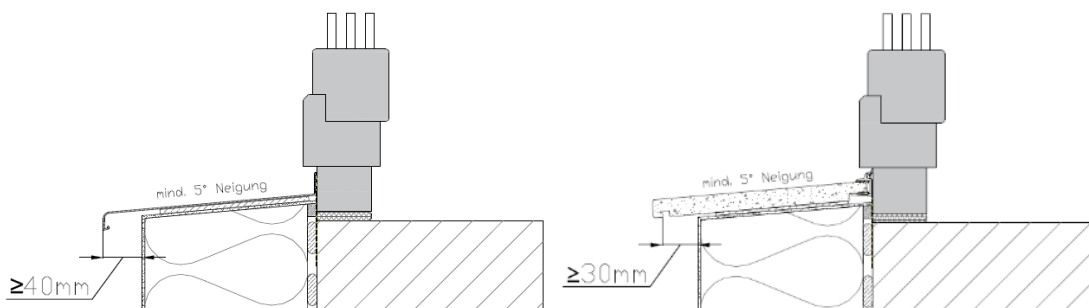
Abbildung 6: schematische Darstellung des Fensterbankvorsprungs bei einer Aluminium- und einer Steinfensterbank
