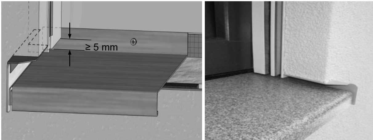
Abbildung 21: eingeputzte Sonnenschutzführungsschiene mit ausgeklinktem Endprofil
