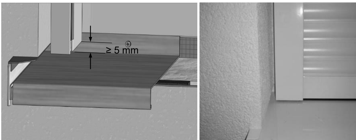
Abbildung 22: nachträglich montierte vorgesetzte Sonnenschutzschiene
