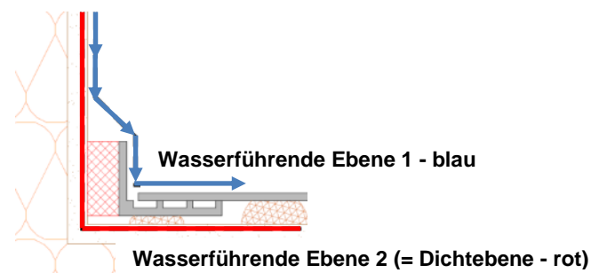
Abbildung 4: Beispiel für den Anschluss der Fensterbank an die Laibung mit zwei wasserführenden Ebenen (Ebene 1 entspricht der Fensterbank; Ebene 2 entspricht der wannenförmigen Abdichtung)
