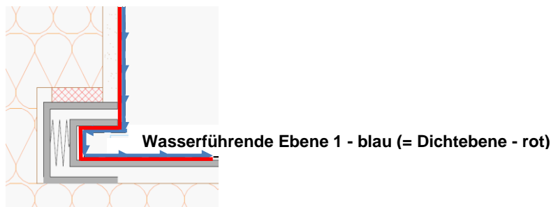
Abbildung 3: Beispiel mit einer wasserführenden Ebene (= Dichtebene)
