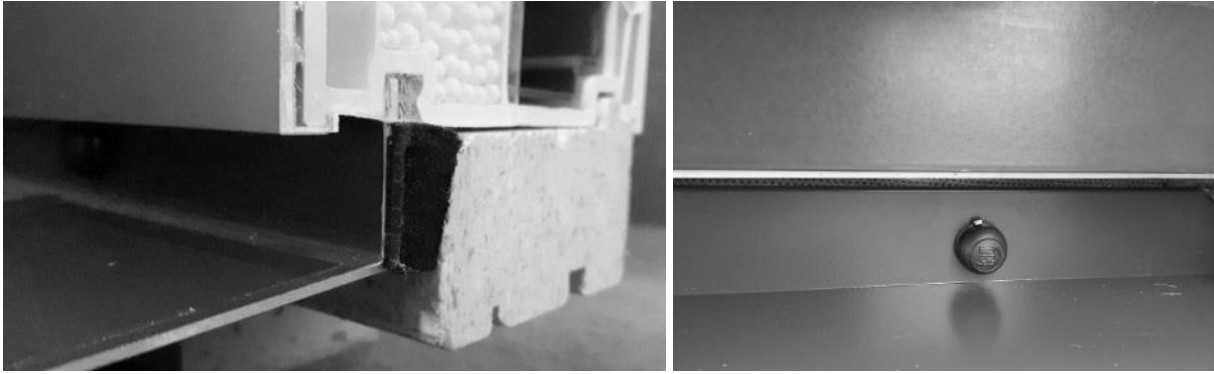
Abbildung 10: Am Fensterbankanschlussprofil des Fensters befestigte und mittels Fugendichtband angedichtete Fensterbank, die hinter die wasserführende Ebene des Fensterrahmens greift.
