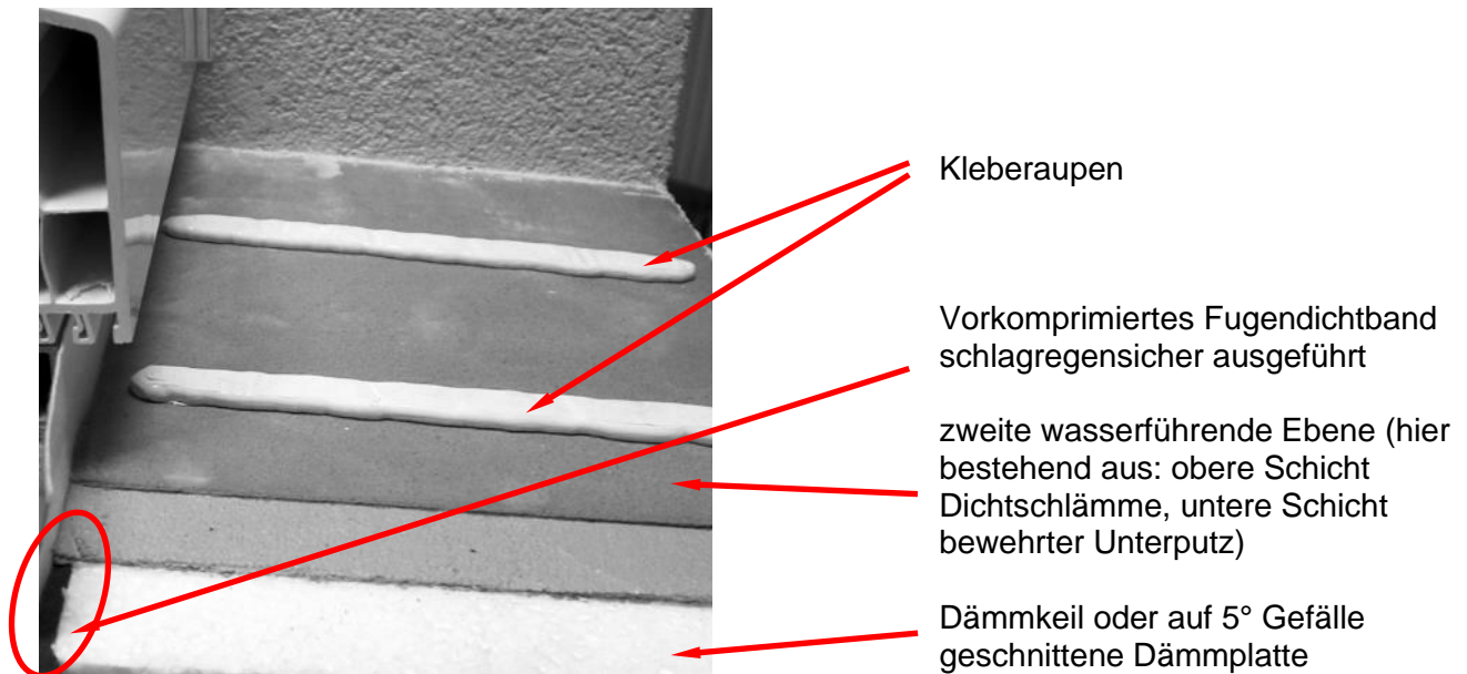
Abbildung 9: Kleberaupen auf zweiter Dichtebene, auf denen die Fensterbank verklebt wird. Die dabei entstehenden Hohlräume zwischen den Kleberaupen sind zulässig. Der Anschluss des Dämmstoffkeils/Fassadenplatte an das Fensterbankanschlussprofil erfolgt mittels vorkomprimierten Fugendichtband.
