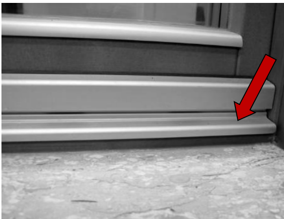
Abbildung 11: Ausführung mit Regenschiene und Wetterschenkel bei stumpfer Montage der Fensterbank an den Fensterrahmen
